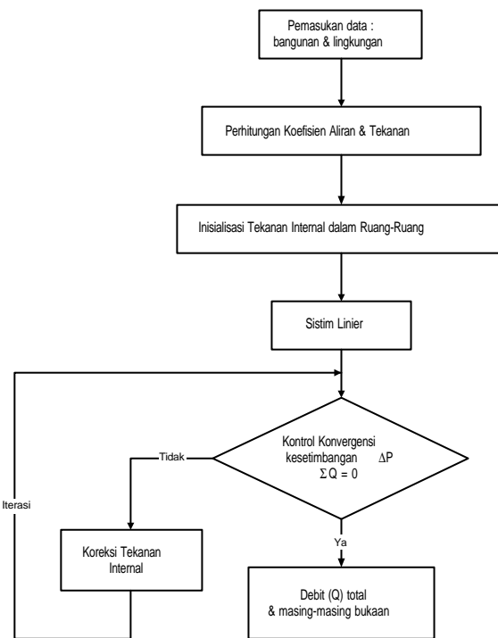
Gambar 1. Diagram alir (flowchart) prosedur perhitungan pada program Ventila.1.0
